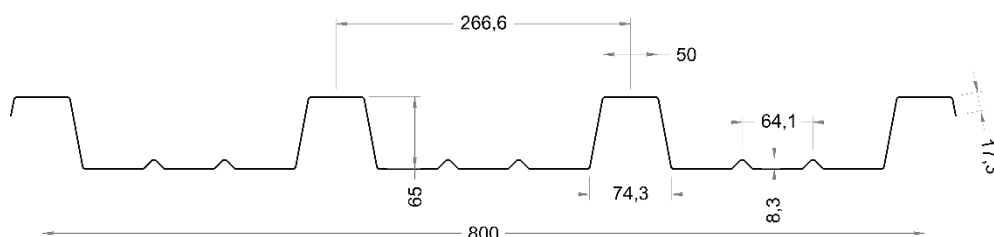
MONTAGEM COBERTURA
