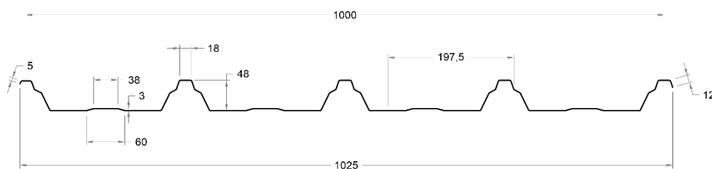
MONTAGEM COBERTURA
