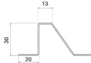
PRI.030 Perfil de listón inclinado 30 mm
