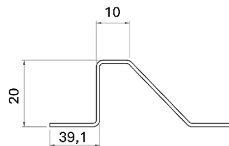
PRI.020 Perfil de listón inclinado 20 mm
