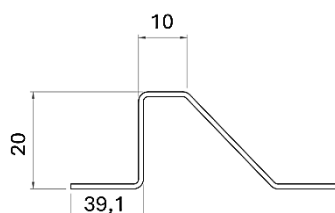
PRI.020 Perfil Ripa Inclinada 20 mm
