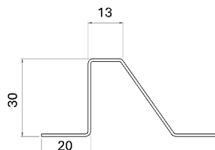
PRI.030 Perfil Ripa Inclinada 30 mm
