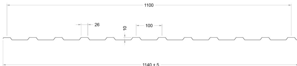
MONTAGEM COBERTURA
